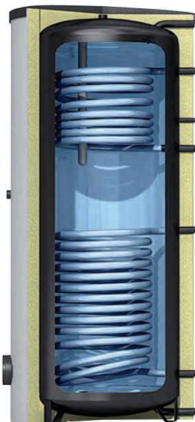
Typ RS-2 mit zwei eingebauten Glattrohrwärmetauschern
