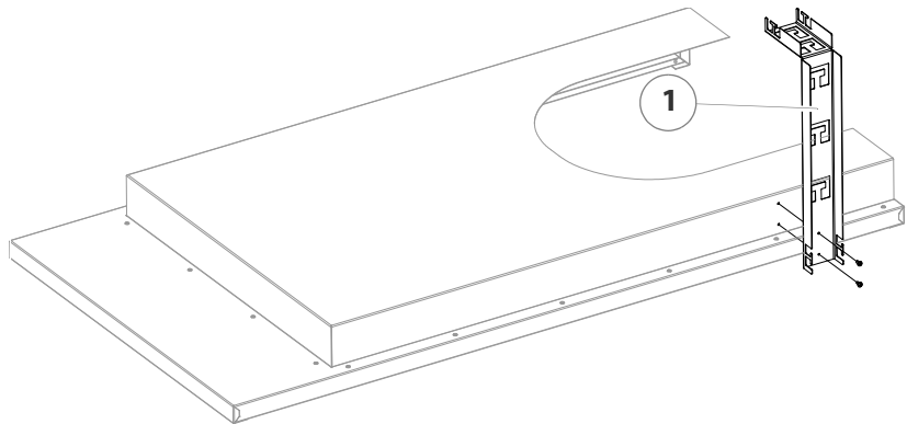
Abbildung 4/64 - Kabelkanal montieren
