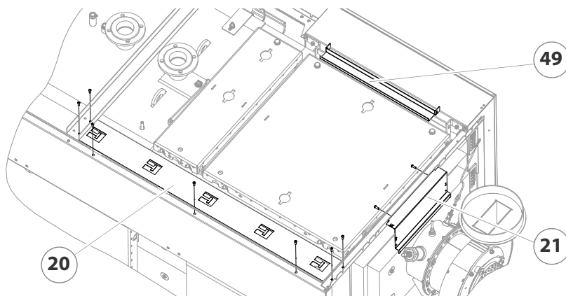
Abbildung 4/26 - Verkleidungsbleche montieren
