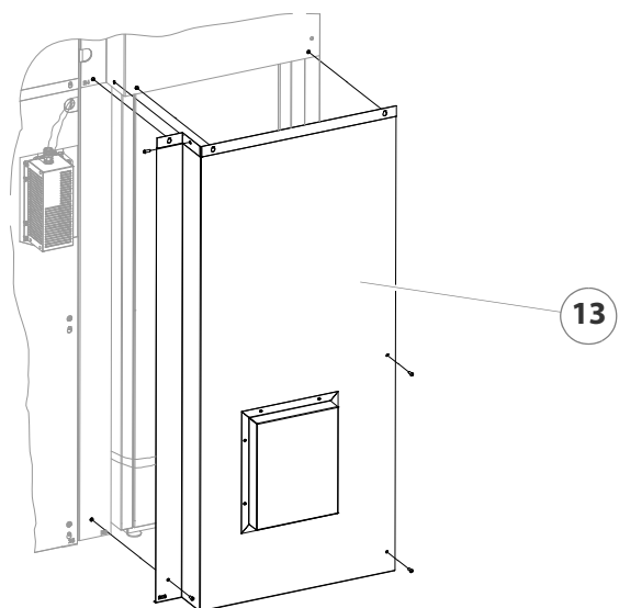
Abbildung 4/61 - Rückseitenverkleidung Feinstaubabscheider montieren
