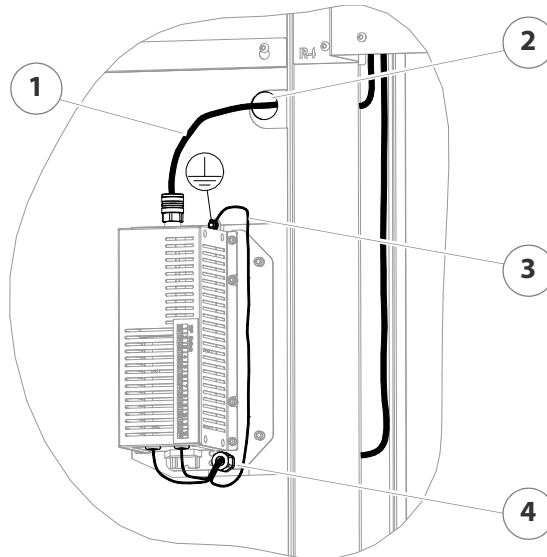
Abbildung 4/52 - Kabel verlegen
