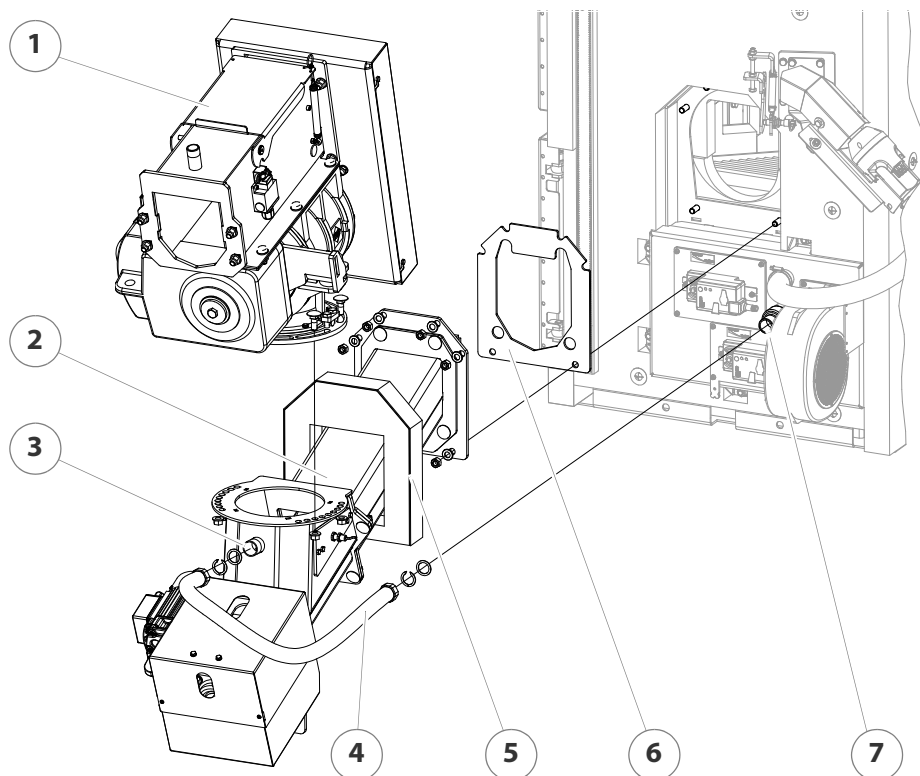
Abbildung 4/14 - Beschickung VBZ 160 montieren
