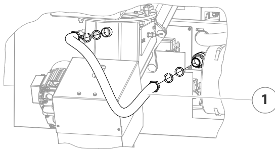
Abbildung 7/24 - Druckausgleichsschlauch reinigen
