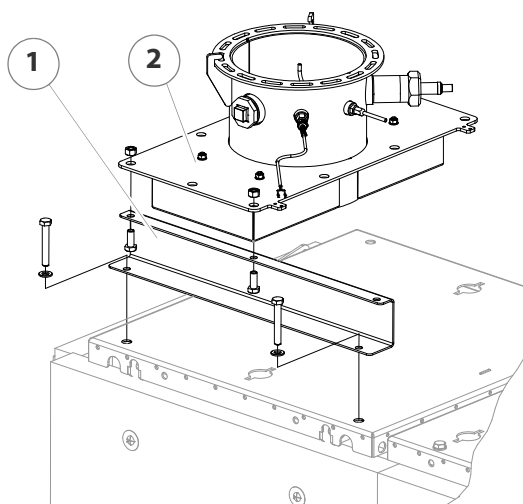
Abbildung 4/11 - Abgasgehäuse demontieren
