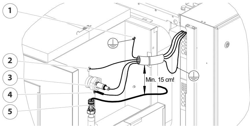
Abbildung 4/49 - Abgasfühler, Lambda-Sonde und Unterdruckschlauch montieren
