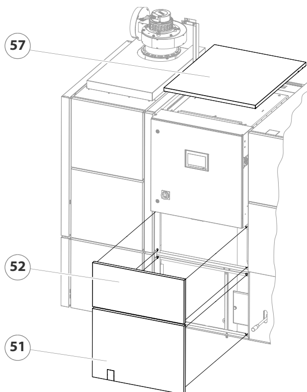
Abbildung 4/66 - Kesselverkleidung montieren
