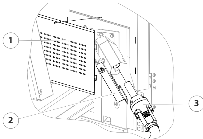
Abbildung 7/21 - Anzündgebläse ausbauen
