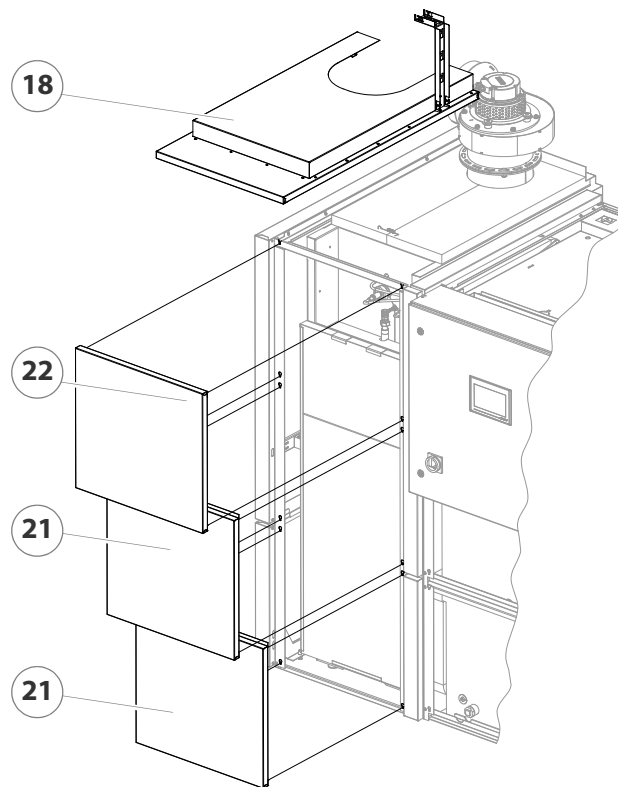
Abbildung 4/65 - Seitenverkleidung Feinstaubabscheider montieren
