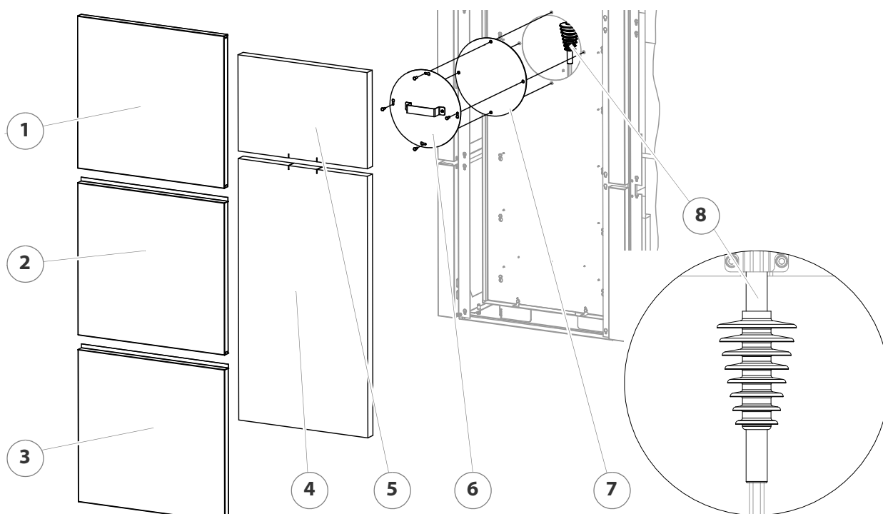
Abbildung 7/3 - Isolator reinigen
