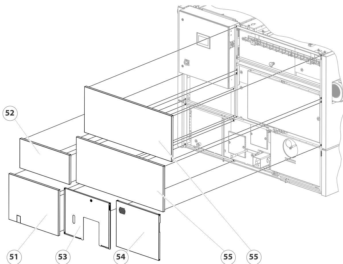
Abbildung 4/31 - Frontverkleidung montieren
