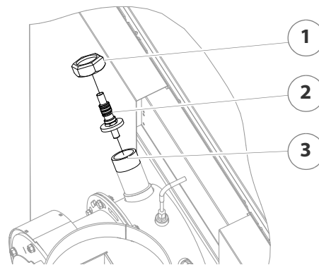
Abbildung 7/17 - Lambda-Sonde reinigen
