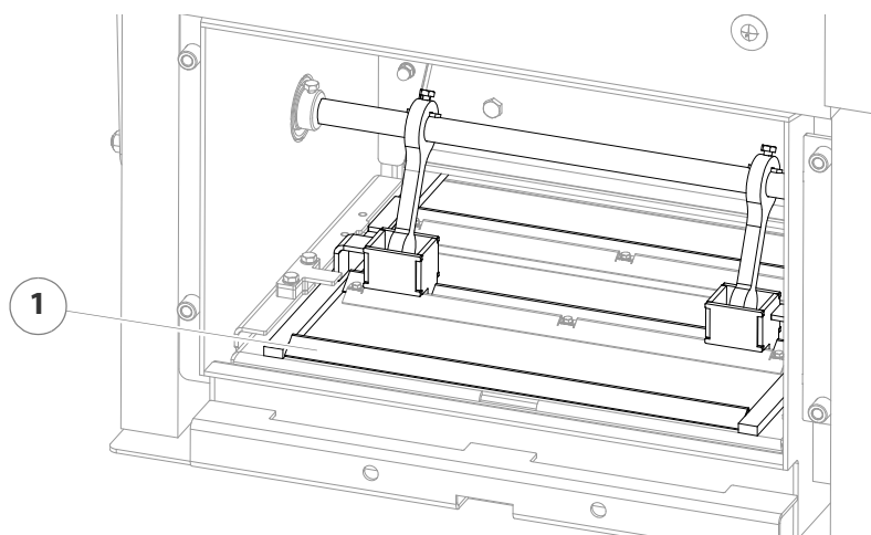
Abbildung 4/39 - Ascheschubboden einstellen
