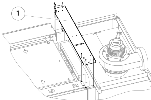
Abbildung 4/59 - Obere Abdeckung montieren
