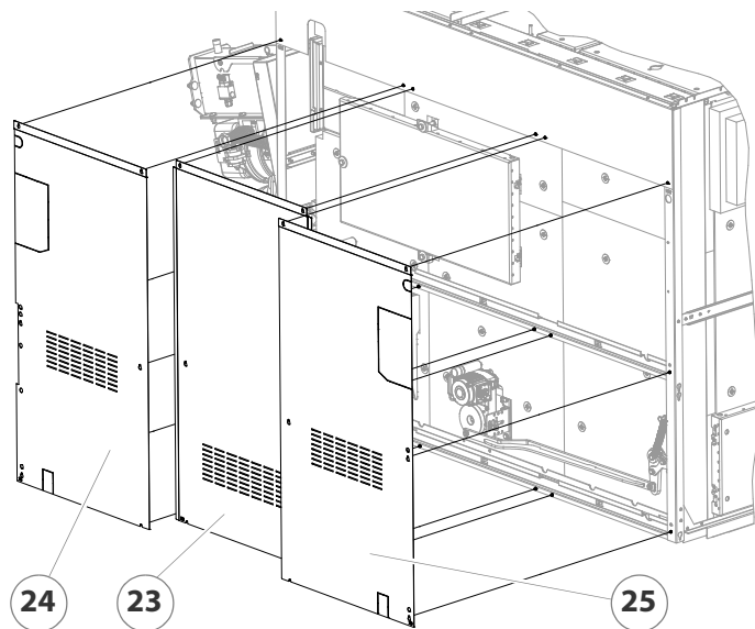
Abbildung 4/28 - Rückseitenverkleidung montieren
