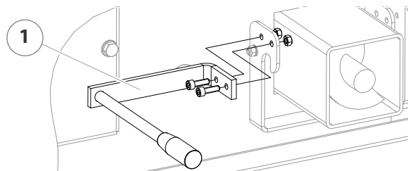
Abbildung 4/13 - Spanngriff montieren
