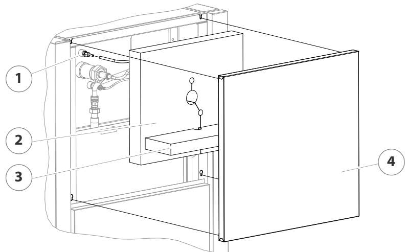
Abbildung 7/16 - Unterdruckrohr reinigen
