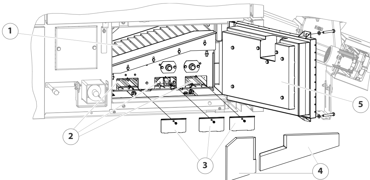
Abbildung 7/5 - Stufenrost reinigen
