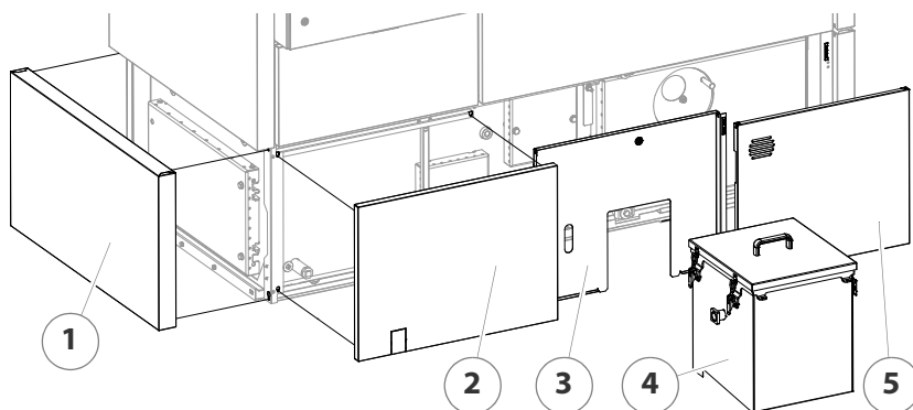
Abbildung 7/25 - Verkleidung demontieren
