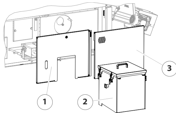
Abbildung 7/4 - Verkleidung demontieren
