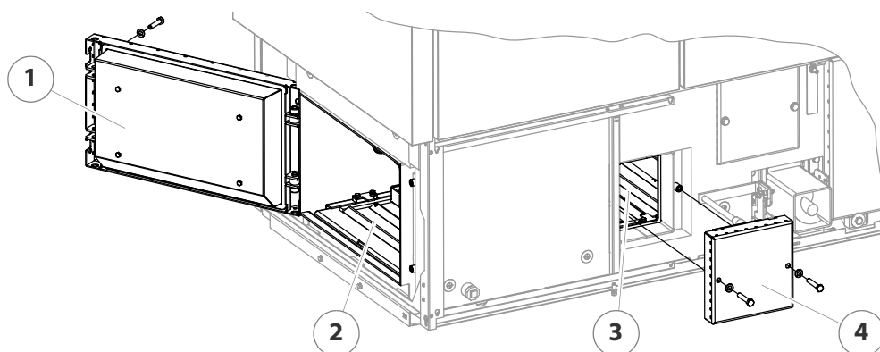
Abbildung 7/26 - Flugaschenbereich reinigen
