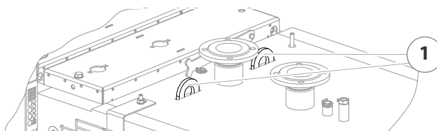
Abbildung 4/7 - Kranösen
