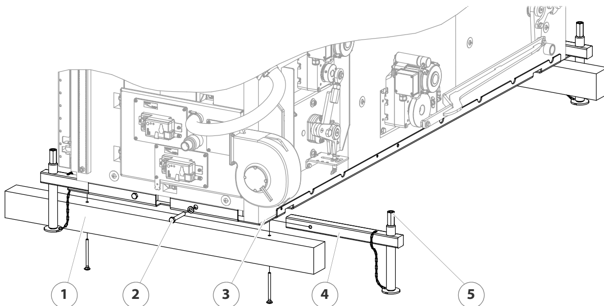
Abbildung 4/8 - Montagehilfe
