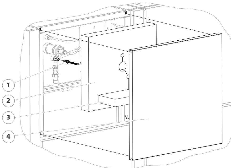
Abbildung 7/20 - Lambda-Sonde reinigen
