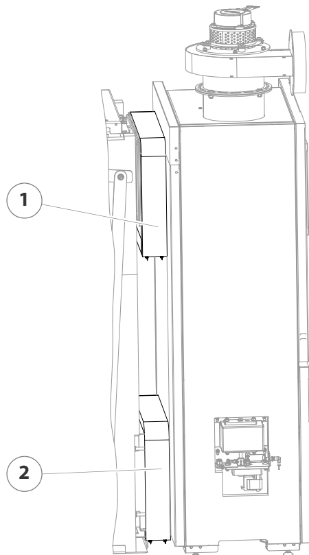
Abbildung 4/48 - Dämmungsmanschetten montieren
