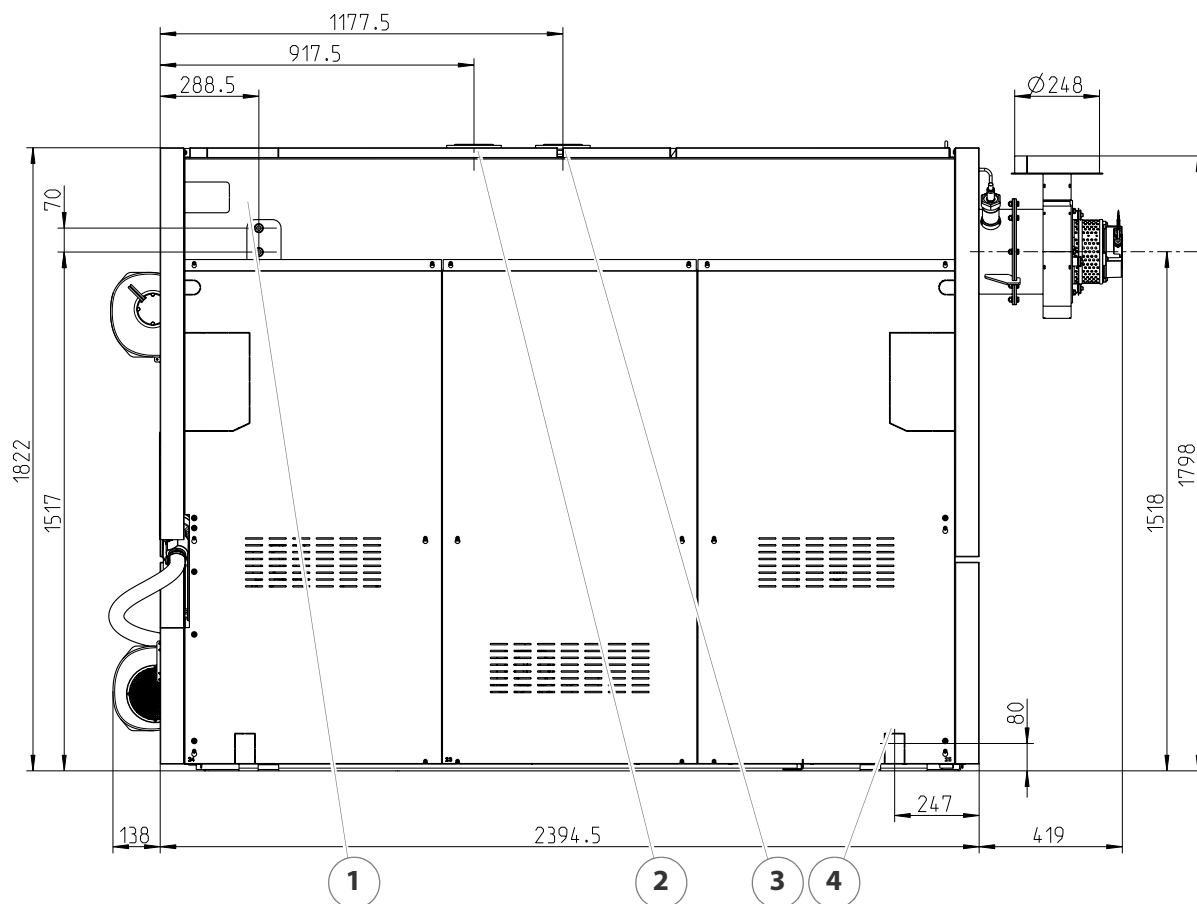
Abbildung 4/1 - Abmessungen Rückseite HDG M150 - 240 (ohne Abscheider)
