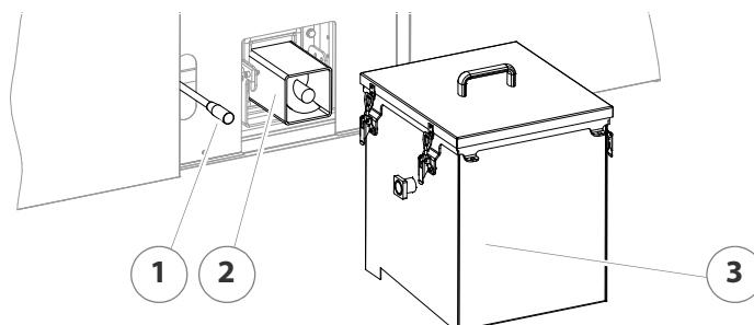
Abbildung 4/34 - Aschenbehälter montieren
