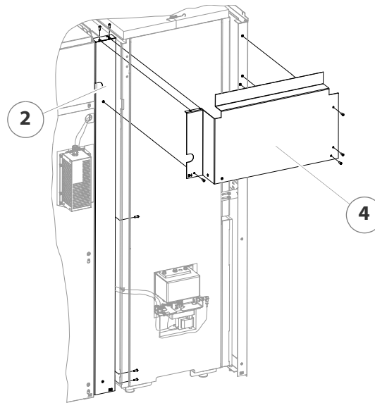
Abbildung 4/58 - Verkleidung montieren
