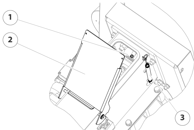
Abbildung 7/11 - Abwurfkopf schmieren
