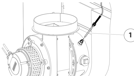
Abbildung 7/19 - Lambda-Sonde reinigen
