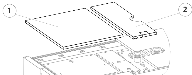
Abbildung 7/12 - Verkleidung demontieren
