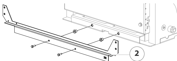
Abbildung 4/38 - Querträger unten montieren
