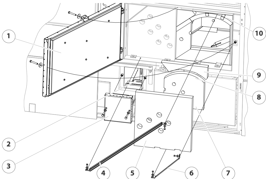
Abbildung 7/7 - Verkleidung demontieren
