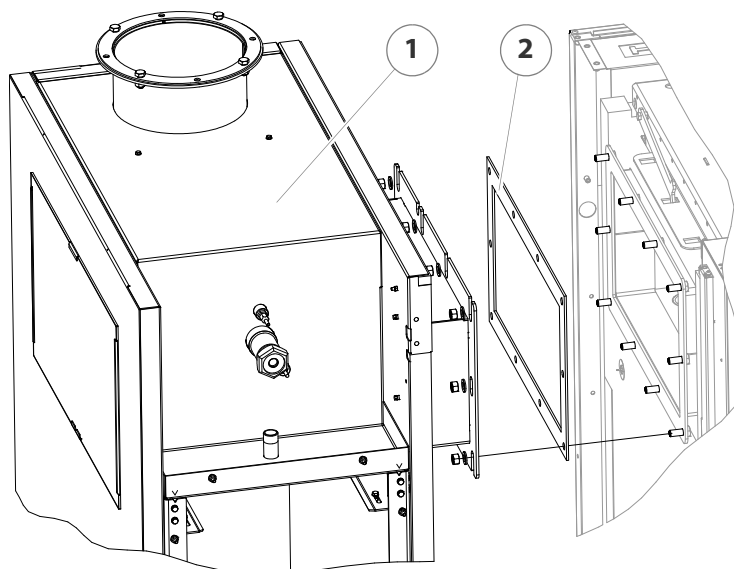
Abbildung 4/40 - Filtergehäuse oben am Kessel montieren
