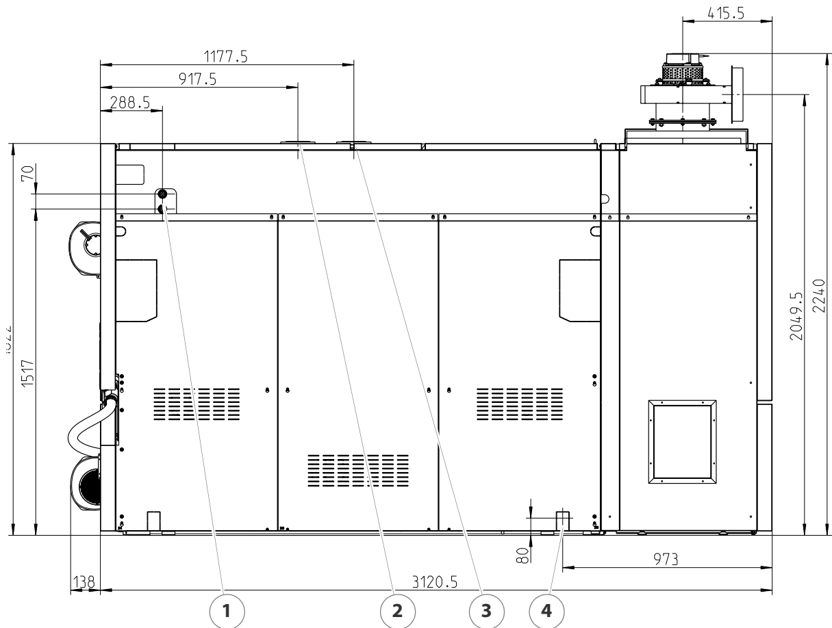
Abbildung 4/2 - Abmessungen Rückseite HDG M175E - 240E (mit Abscheider)
