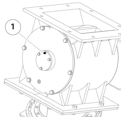
Abbildung 7/10 - Zellenrad schmieren (VBZ 200)
