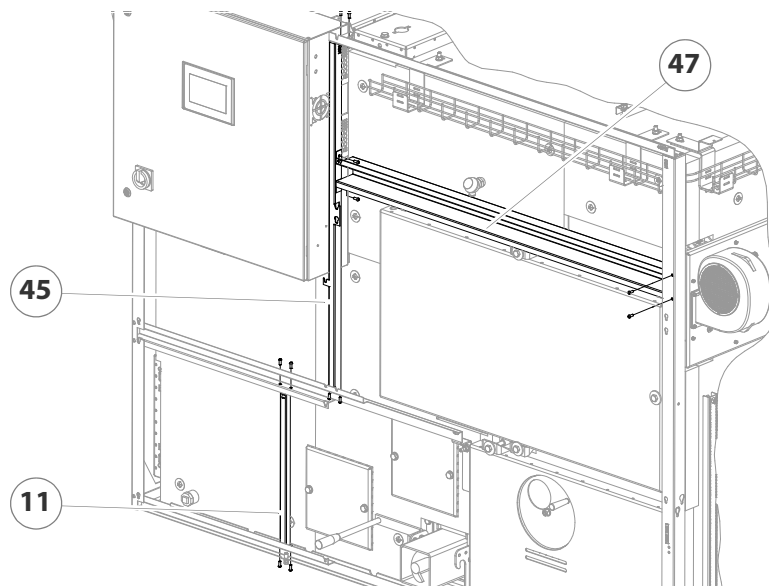
Abbildung 4/21 - Mittelträger montieren
