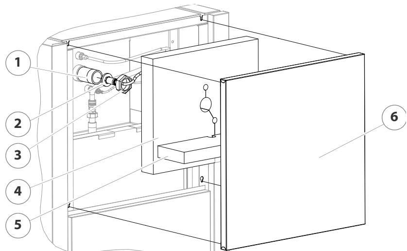
Abbildung 7/18 - Lambda-Sonde reinigen
