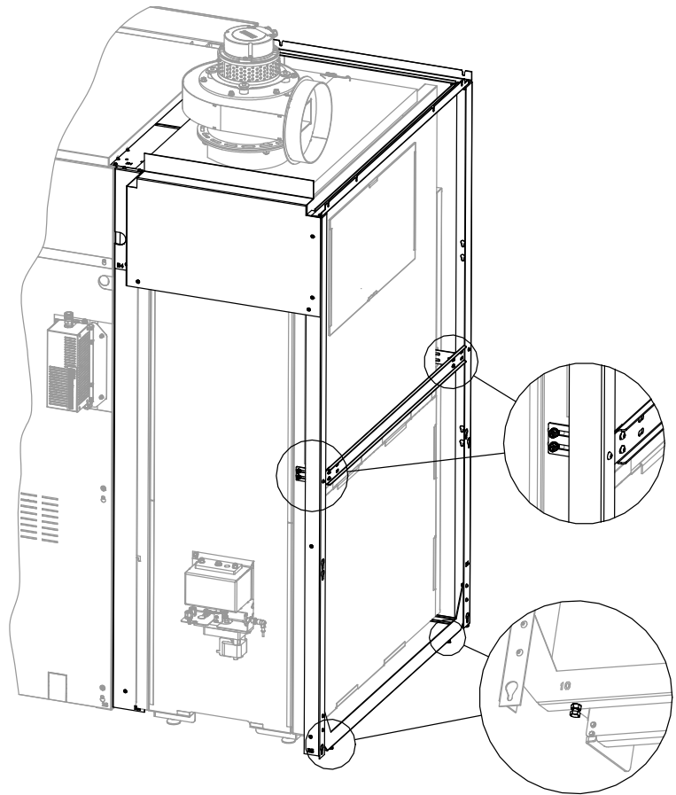
Abbildung 4/60 - Verkleidung ausrichten
