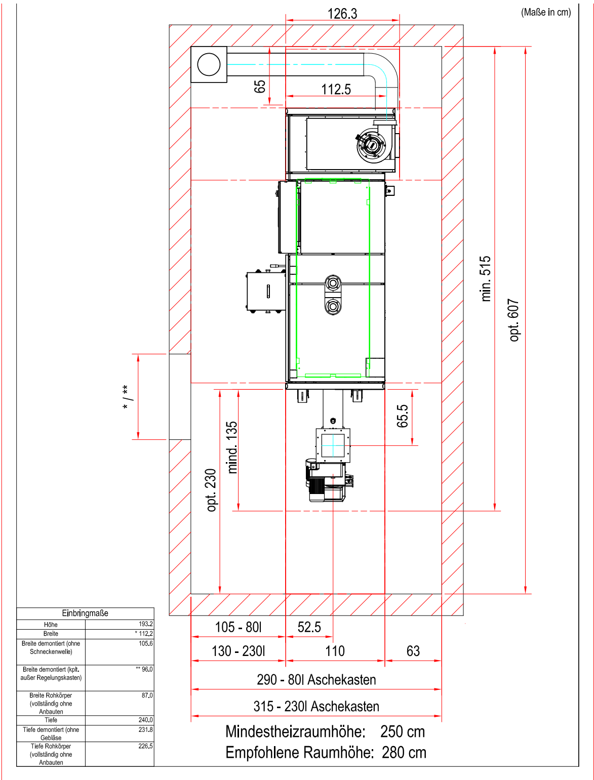
Abbildung 4/5 - Erforderliche Raumgrößen (mit Feinstaubabscheider und VBZ 200)
