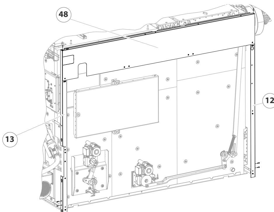
Abbildung 4/22 - Eckträger Rückseite montieren
