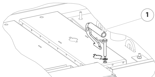
Abbildung 7/13 - Verkleidung demontieren
